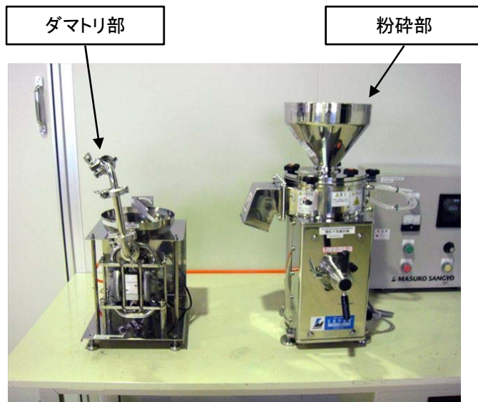
微粒子用摩砕機の概要
