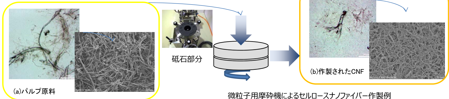
微粒子用摩砕機の概要
