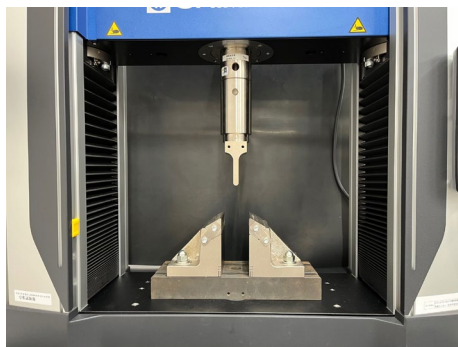
曲げ試験用治具
