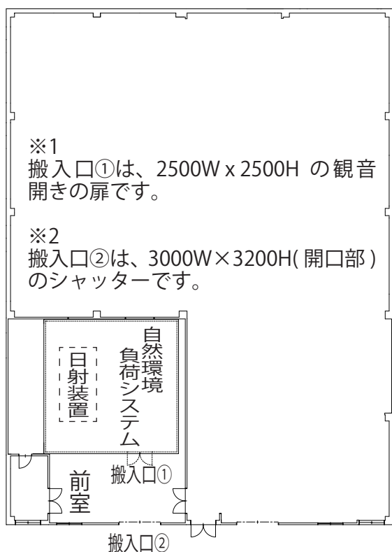
搬入口詳細図
