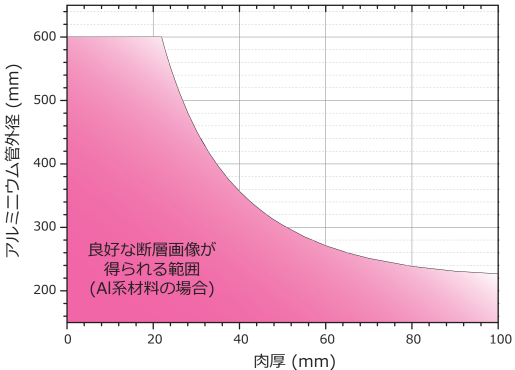
CTスキャンが可能なアルミニウム管の肉厚及び外径の範囲 (曲線はX線透過距離の限界を示す)
