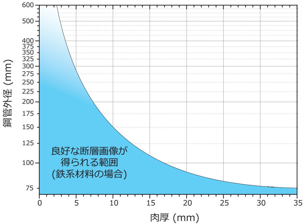
CTスキャンが可能な鋼管の肉厚及び外径の範囲 (曲線はX線透過距離の限界を示す)
