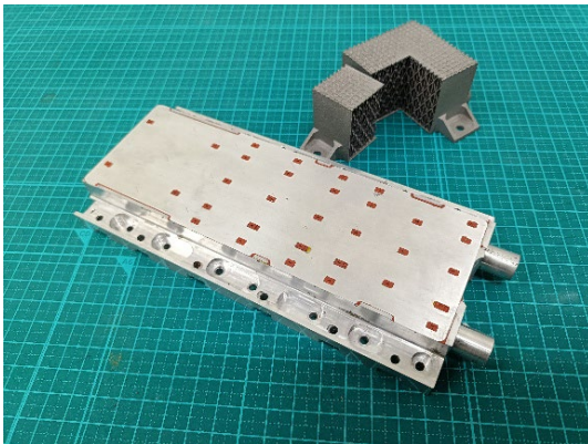
宇宙機向け構造一体型蓄熱デバイス
