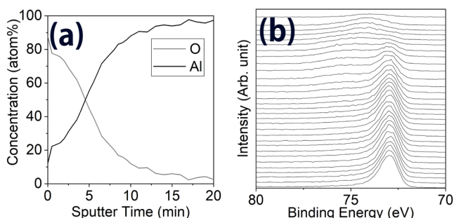
アルミ表面の酸化膜の深さ方向分析結果 (a) プロファイル、(b) Al 2p ナROWSペクトル
