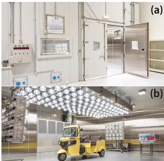
(a) 試験室の外観写真
